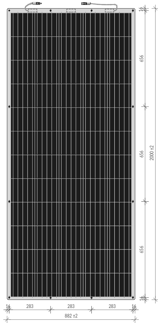
Maßstab 1:15 Modulabmessungen
